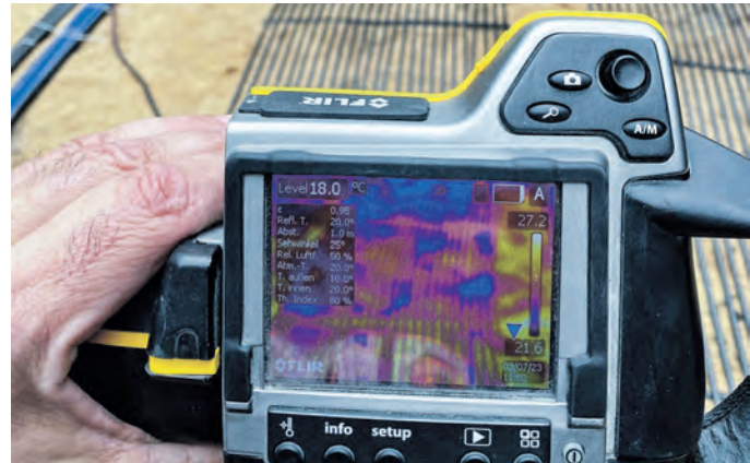
Das ganzjährig konstante Temperaturniveau im Boden – zu erkennen mit der Wärmebildkamera – ermöglicht ein effizientes Heizen.
